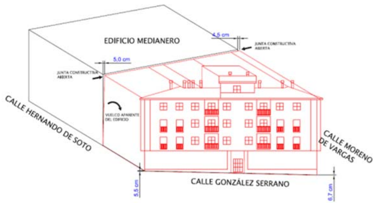
Levantamiento geométrico inicial y toma de datos
