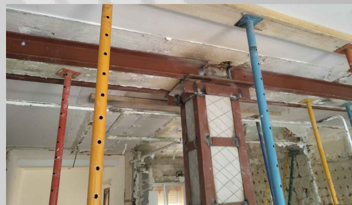
Refuerzo metálico de la viga
